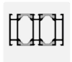
⊕ Rahmenverbreiterung | 44 mm
